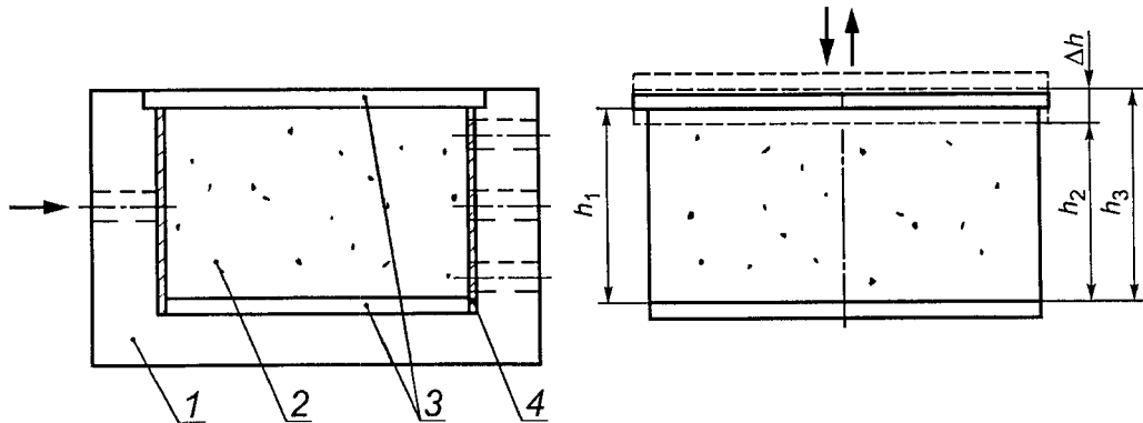
Рисунок 2. Схема приспособления для испытания прямых монтажных швов на деформационную устойчивость
