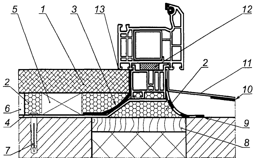
Рисунок А.3. Узел бокового примыкания оконного блока к проему с четвертью слоистой стены из кирпича с эффективным утеплителем и отделкой внутреннего откоса штукатурным раствором
