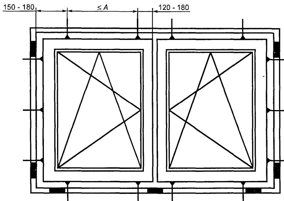
а) Оконный блок с ветрикальным импостом
